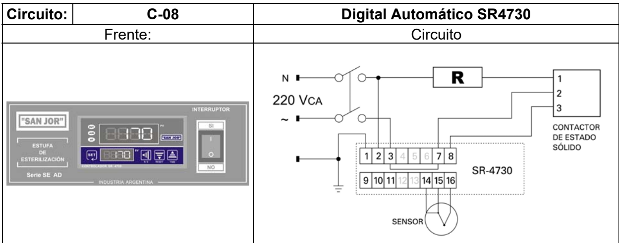
Esquema de Conexión
