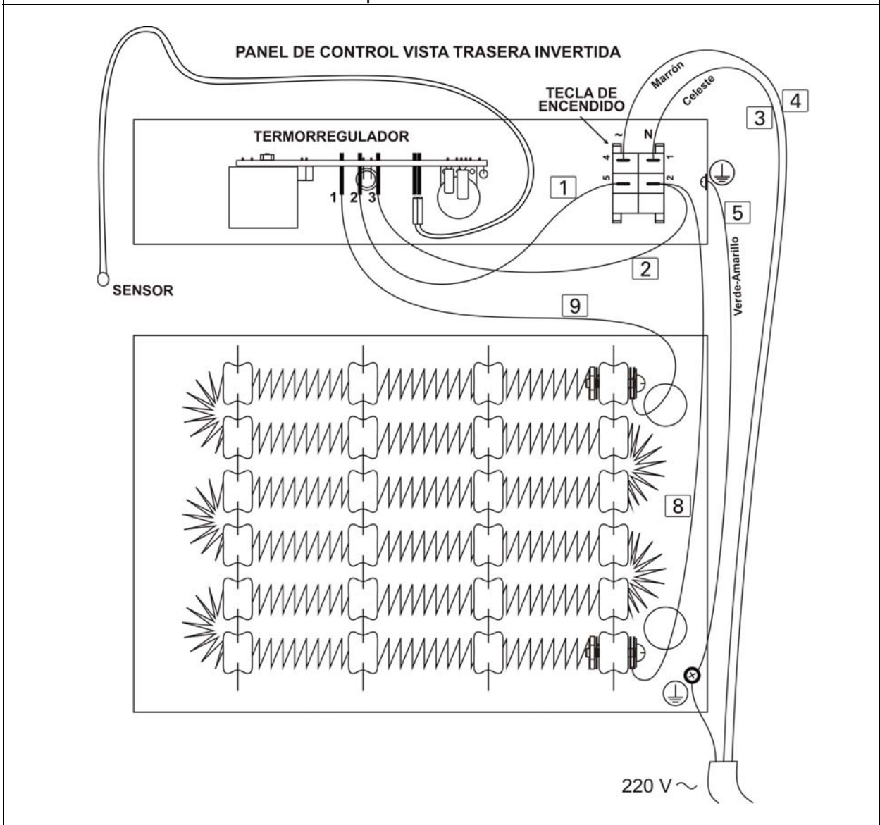
Esquema de Conexión
